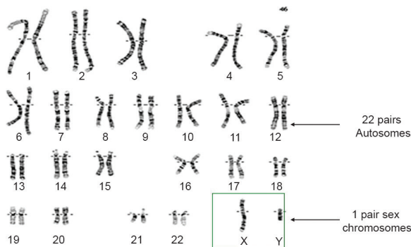
Autosome
