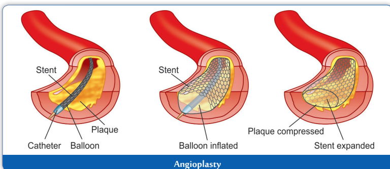
Angioplasty
